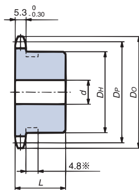
（切削加工规格） 1B型
