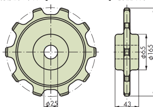
販売終了品【TP-C12724T-IW】（成形品）
