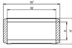
TKA形 A-A断面 (アーム外周側開閉)
