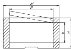
TKC形 A-A断面
