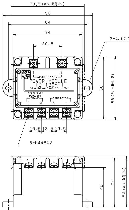
400V 用電源装置 HD-120MH1 寸法図
