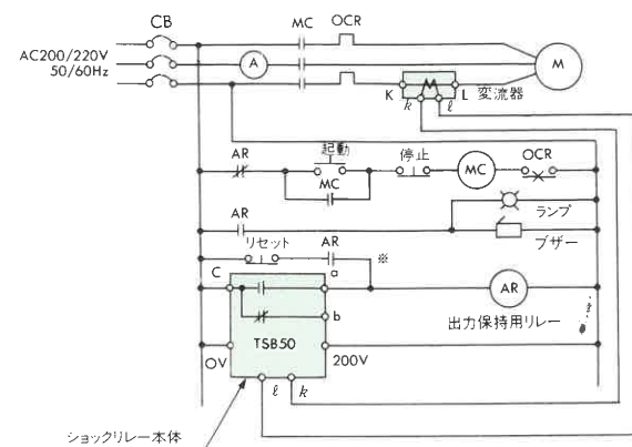
■接続図
