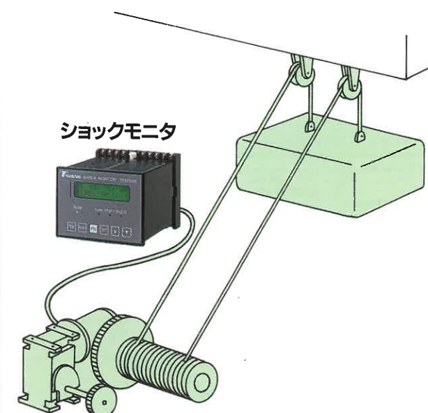
昇降装置
