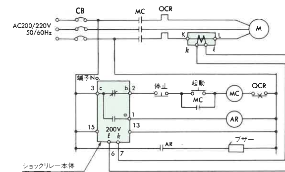
■接続図
