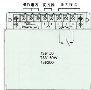
■TSB150, 150W, 200シリーズ共通端子配置
