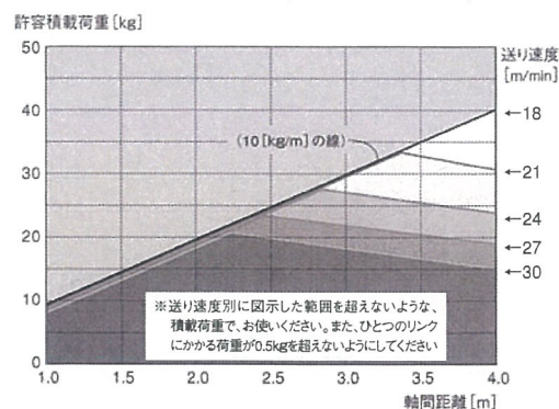
図2. 許容積載荷重線図 (直動式ユニット)
