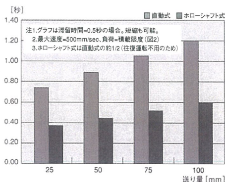
図1. タクトタイム
