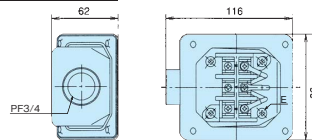
1.5kW～3.7kW
