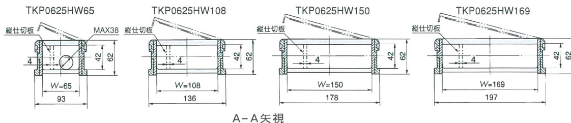
A-A 矢視
