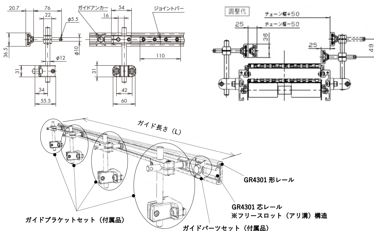
図 4.プロダクトガイド外形寸法
