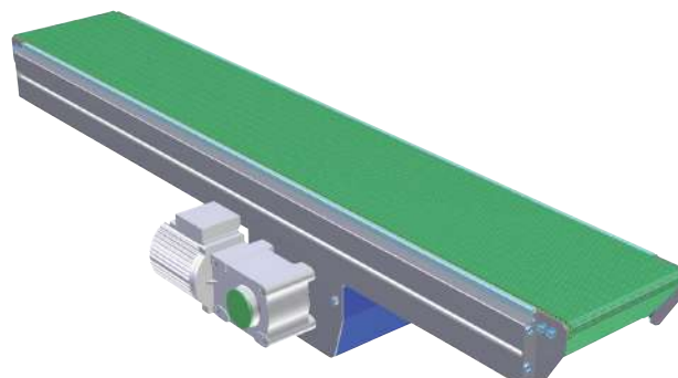
中間駆動(正逆運転可能)
