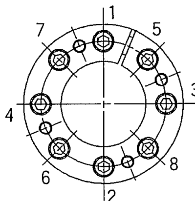
図3 ボルトの締付け順序例
