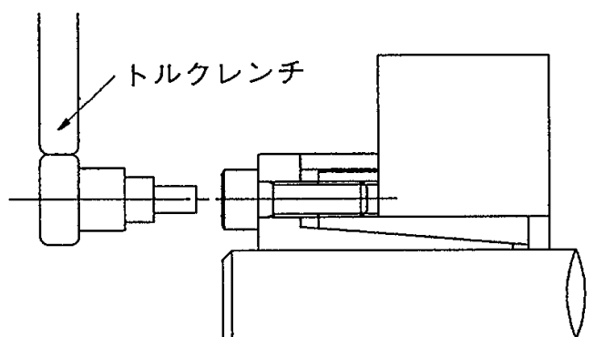
図2 取付け
