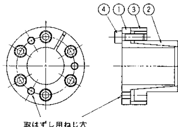
1. インナーリング 3. スペーサ 2. アウターリング 4. 締付ボルト
