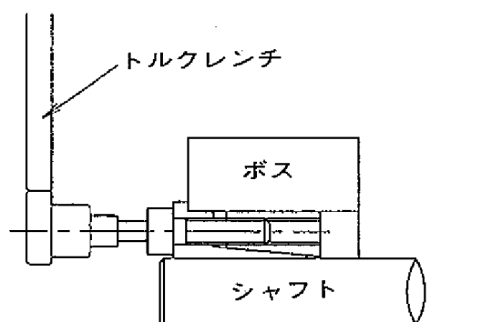
図2 取付け
