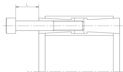
図6 テーパーリングロック解除状態
