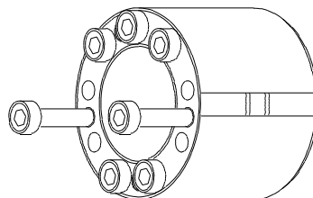
図2 仮組状態
