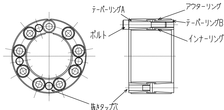
図1 部品名称
