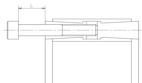
図6 テーパリングロック解除状態
