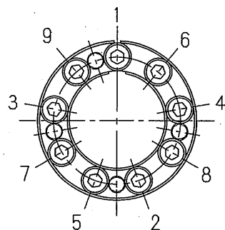
図4 ボルトの締付け順序例
