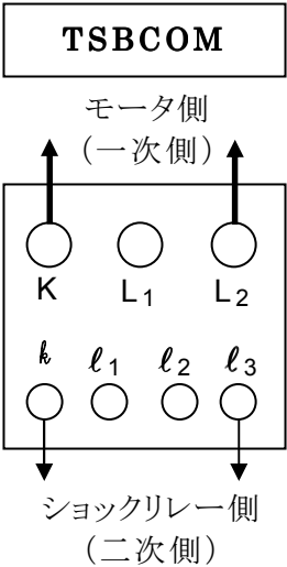
上図はモータ 0.75kW200V の例です。
