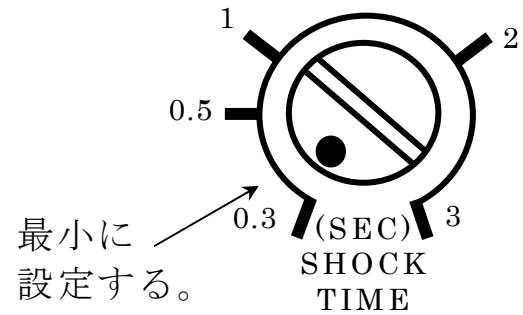
SHOCK TIME 設定ボリューム
