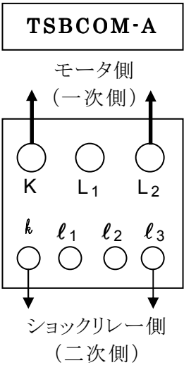
上図はモータ定格電流 0.4A の例です。
