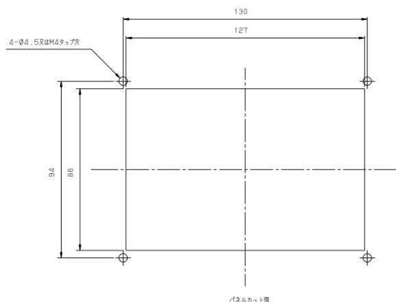
パネルカット図
