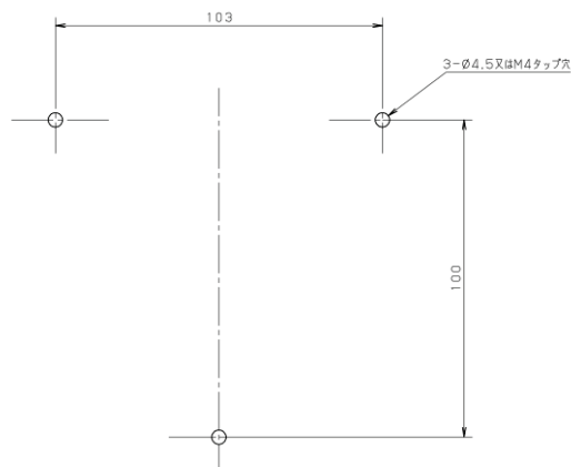
取付けピッチ寸法図
