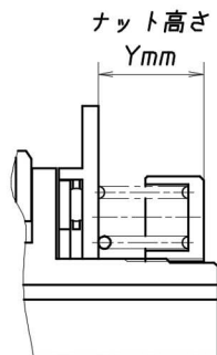
図 10.1. ナット高さ
