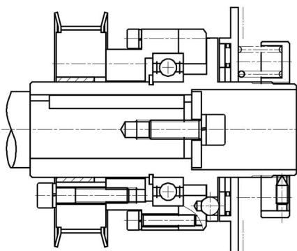
図 5.1. 軸端にタップを加工し、エンドプレートとボルトで固定
