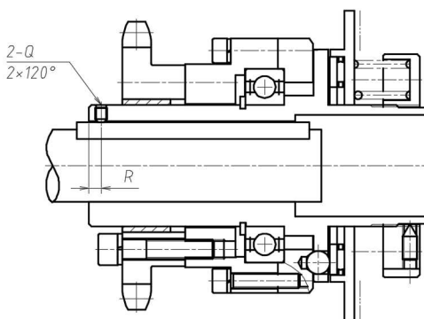
図 5.2. ハブ外周よりタップを加工し、押ネジで固定
