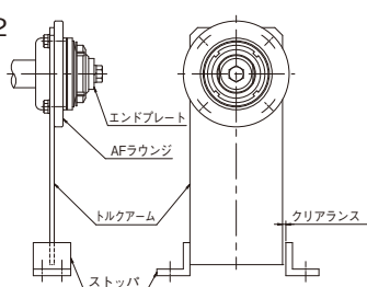
取付例2
