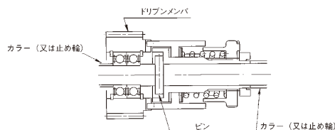
図 3 取付例
