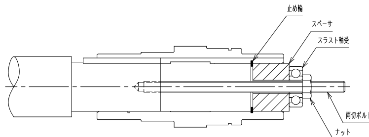
取付治具
