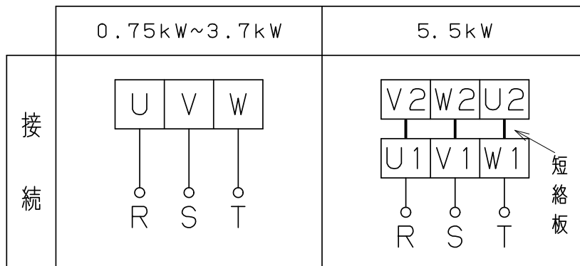
図 6 接続方式
