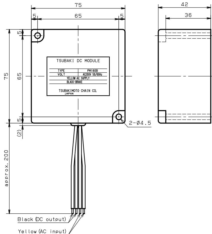
電源装置 PM180B 寸法図
