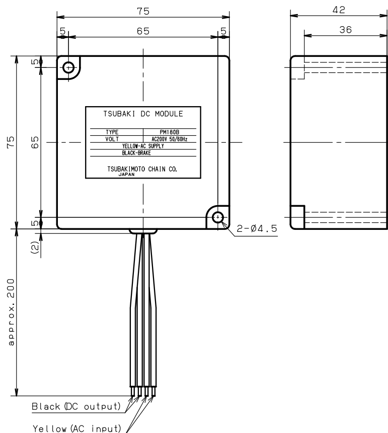
電源装置 PM180B 寸法図
