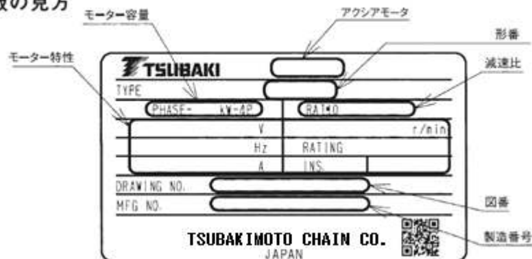
銘板の見方
