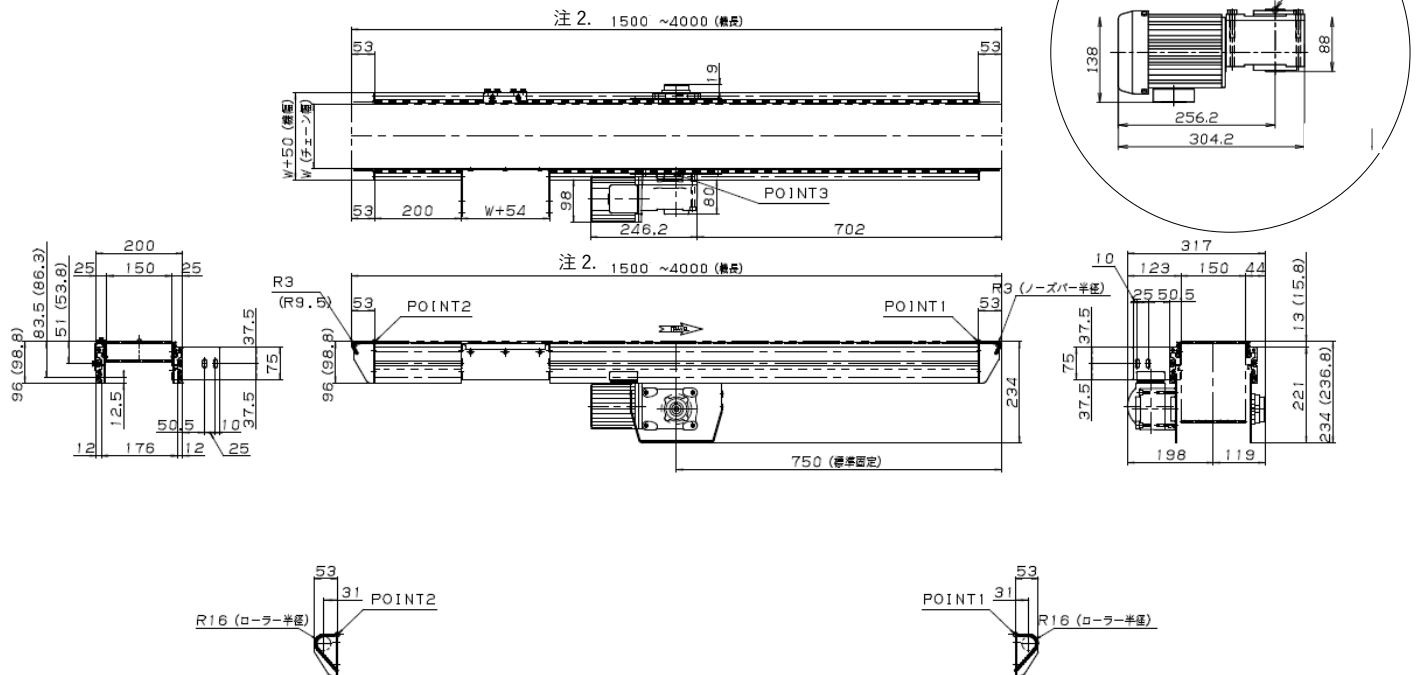
図 1.外形寸法図
