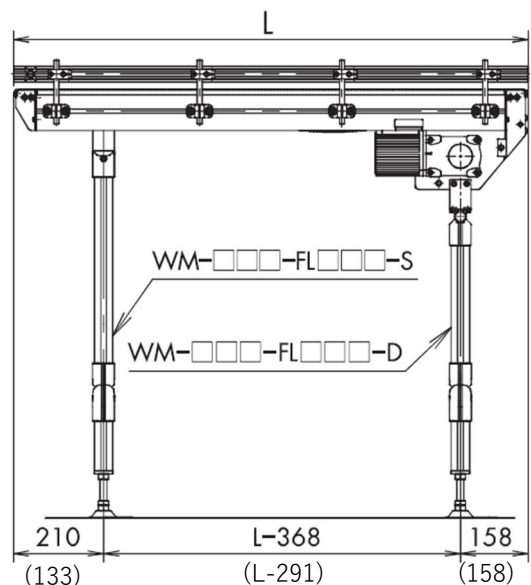
〔駆動下支持（仕様記号：D）1 本、コンベヤフレーム支持（仕様記号：S）1 本〕
