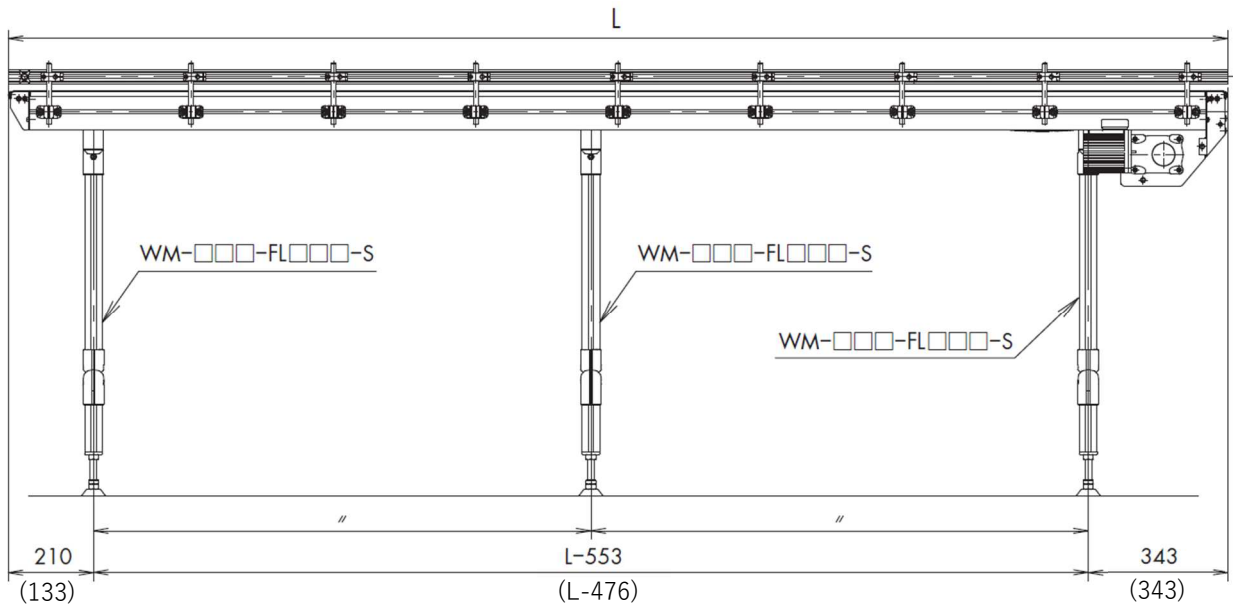
〔コンベヤフレーム支持（仕様記号：S）3 本〕
