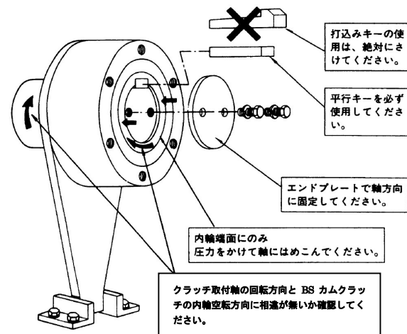
取付手順図
