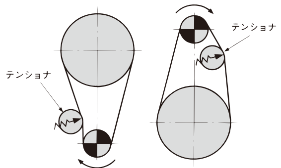
図39. 垂直伝動
