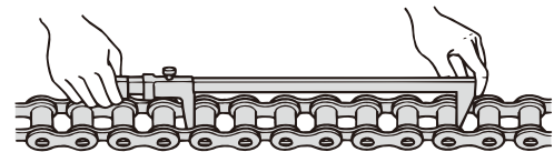
ノギスにて6リンク測定のところ
