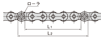
図45. 長さの測定
