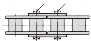
図1. リベット形ローラチェーン
