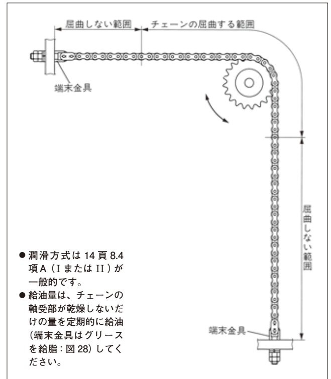
図 27. 給油する箇所
