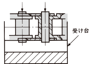
図 12. プラコンビチェーンを 受け台にセット
