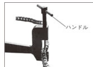
図7. ローラチェーンの支持 （RS-CS-A形チェーンスクリュ）
