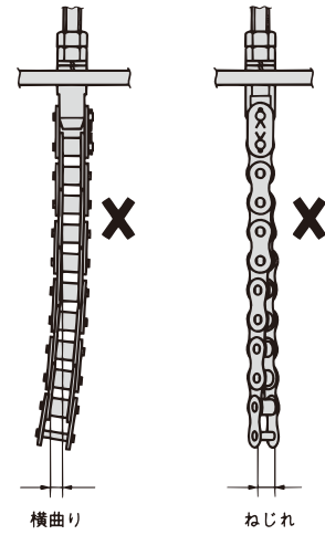
図46. ローラチェーンの横曲りとねじれ
