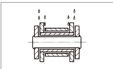
図 26. 給油の位置
