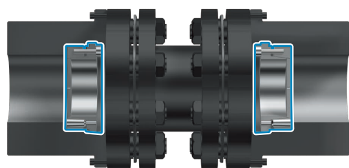
パワーロック 内側取付
