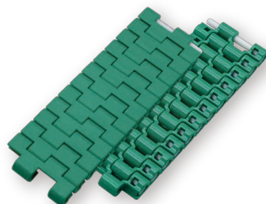
WT0705-M形 固定幅タイプ (チェーンピッチ7.5mm)
