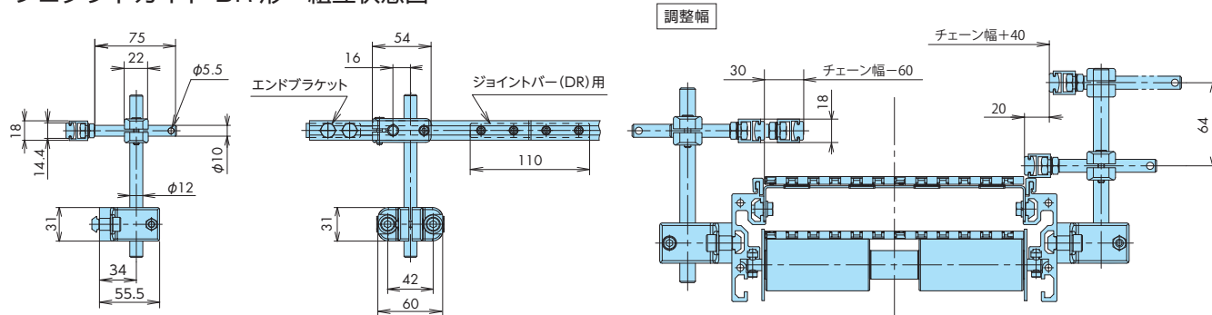
プロダクトガイド DR形 組立状態図
