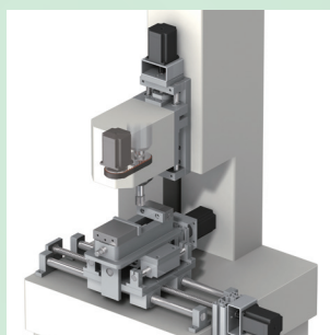
ホーニングマシン
